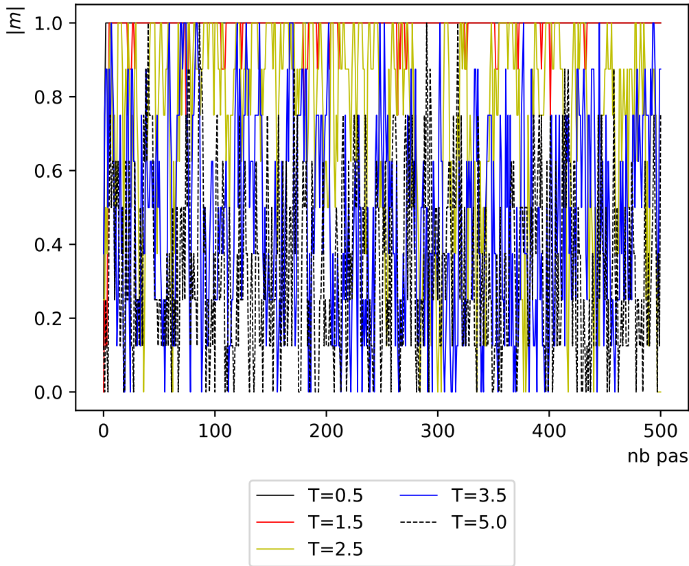
Evolution de l'aimantation sur 500 pas de Monte Carlo, N=4
